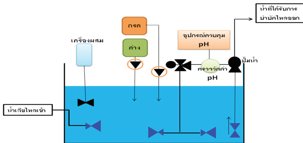
ภาพที่ 10 การทำให้เป็นกลางโดยใช้กรดหรือด่าง
