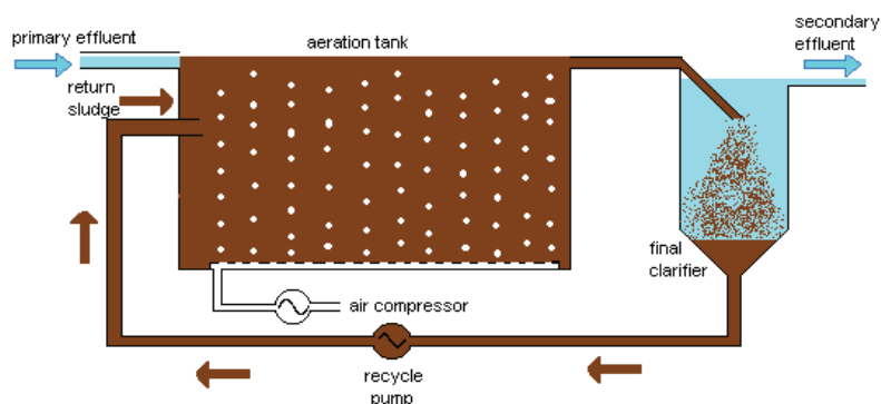
ภาพที่ 14 ระบบบำบัดน้ำเสียแบบแอคติเวตเต็ดสลัดจ์หรือตะกอนเร่ง (Henz et al., 2002)
